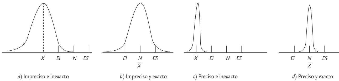
■ FIGURA 11.4 Precisión y exactitud a través de la curva normal.
