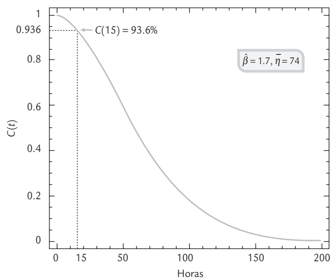
■ FIGURA 13.11 Función de confiabilidad, ejemplo 13.6.
